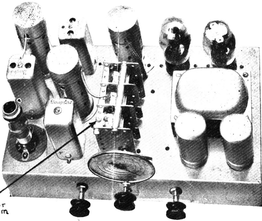
Chassis armado visto de arriba
