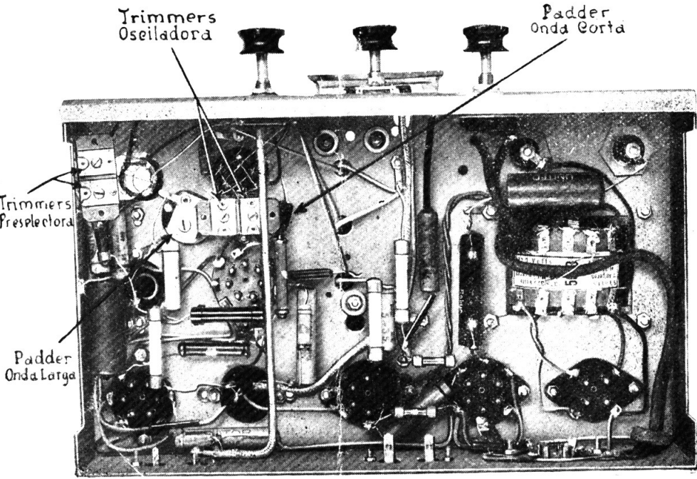
Chassis armado visto de abajo
